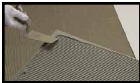
Fig.29 - Applicare l'adesivo con la tecnica della doppia spalmatura e cioè stendendo l'adesivo a letto pieno sul supporto, usando una spatola a denti distanziati tra loro di almeno 6 mm (ad esempio Raimondi art.138HFV6 ). Quindi applicare l'adesivo anche sul retro della lastra, utilizzando una spatola con denti da 3 mm. Ricordarsi di ripassare l'adesivo sul perimetro della lastra.
